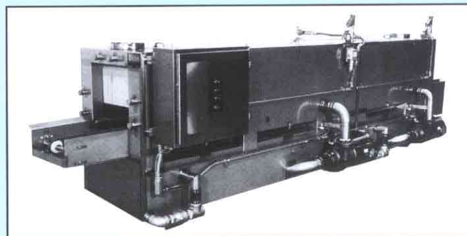
TUNNEL CASE WASHER FOR PLASTIC AND METAL CRATES LAVADORA TIPO TUNEL PARA CANASTAS PLASTICAS Y METALICAS
